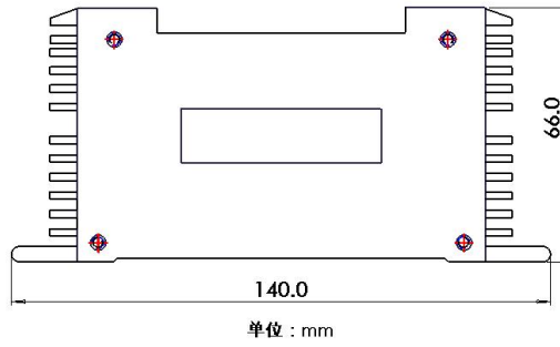
图 8-2 控制器安装尺寸图 2
