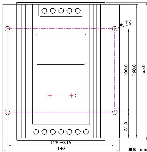
图 8-1 控制器安装尺寸图 1
