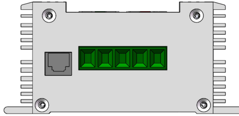
图 2-3 产品上侧连接口图
