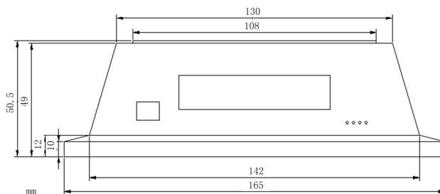
图 8-1 JN-K 系列控制器安装结构示意图一
