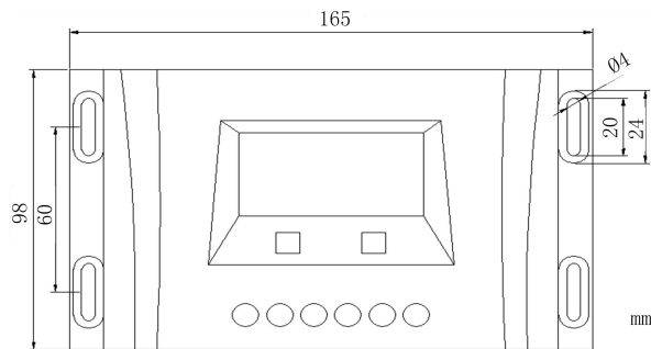
图 8-1 JN-K 系列控制器安装结构示意图一
