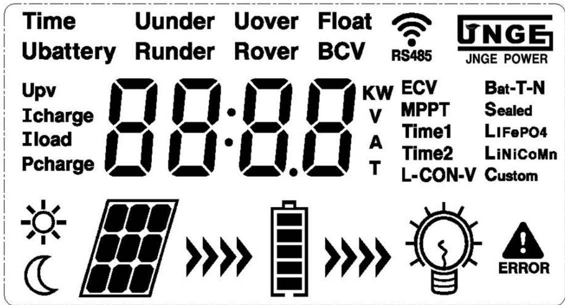
图 4-1 显示屏布局图
