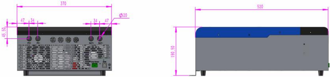
图 8-1 JN-HV2 控制器安装尺寸图(mm)
