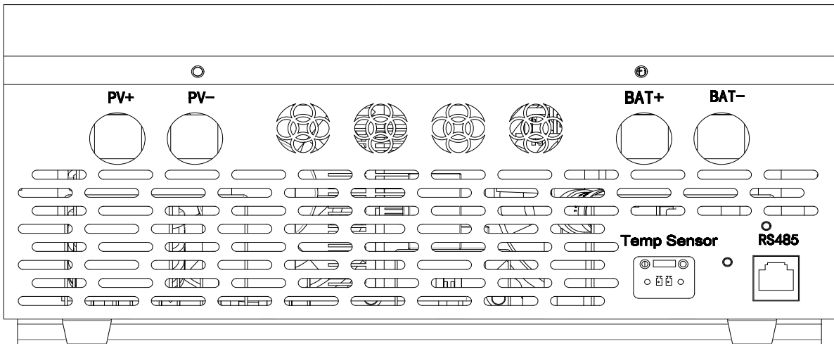
图 2-2 产品接口定义图
